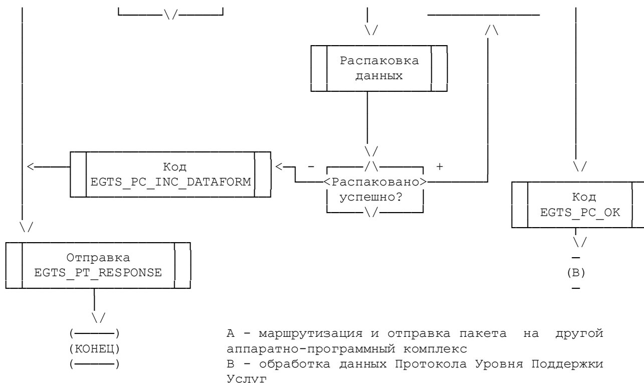
Рисунок 2. Блок-схема алгоритма обработки пакета данных протокола Транспортного уровня при приеме
